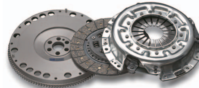
スポーツディスク付KIT ■26000-RB2-1TN
