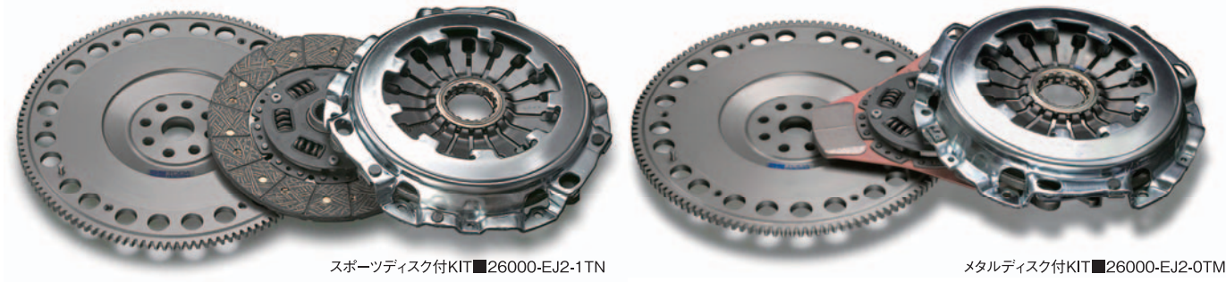
スポーツディスク付KIT ■26000-EJ2-1TN
