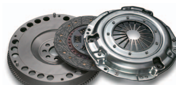
スポーツディスク付KIT ■26000-3SG-02N
