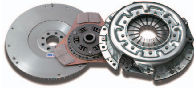
メタルディスク付KIT ■26000-SR2-0TM
