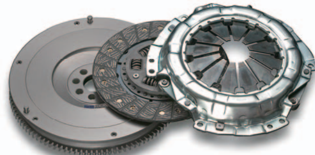
スポーツディスク付KIT ■26000-1ZZ-01N
