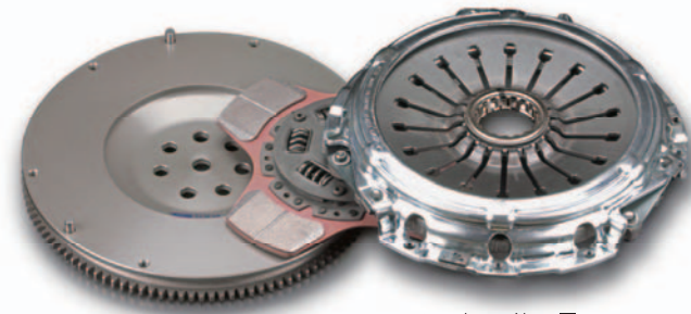
メタルディスク付KIT ■26000-4G6-32M
