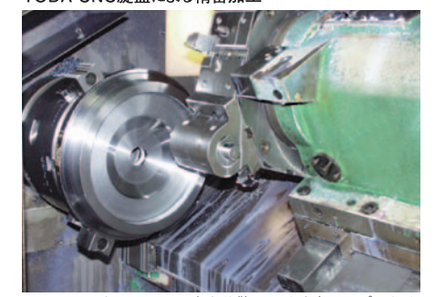
TODAフライホイールは、応力分散による強度アップのため、断面に曲線ラインを多用したオリジナルデザイン。細部にまで正確な加工を必要とするため、CNC旋盤は不可欠です。
