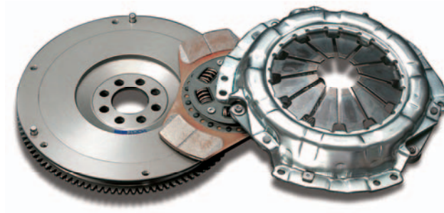
メタルディスク付KIT ■26000-2ZZ-00M
